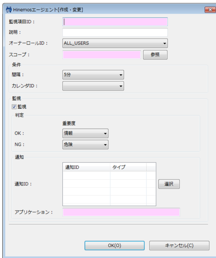
図 7-5 Hinemosエージェント[作成・変更]ダイアログ
